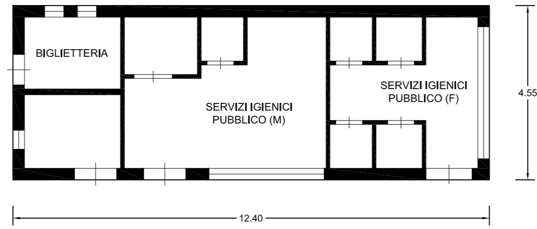
PIANTA LOCALI SERVIZI PUBBLICI SCALA 1:100
